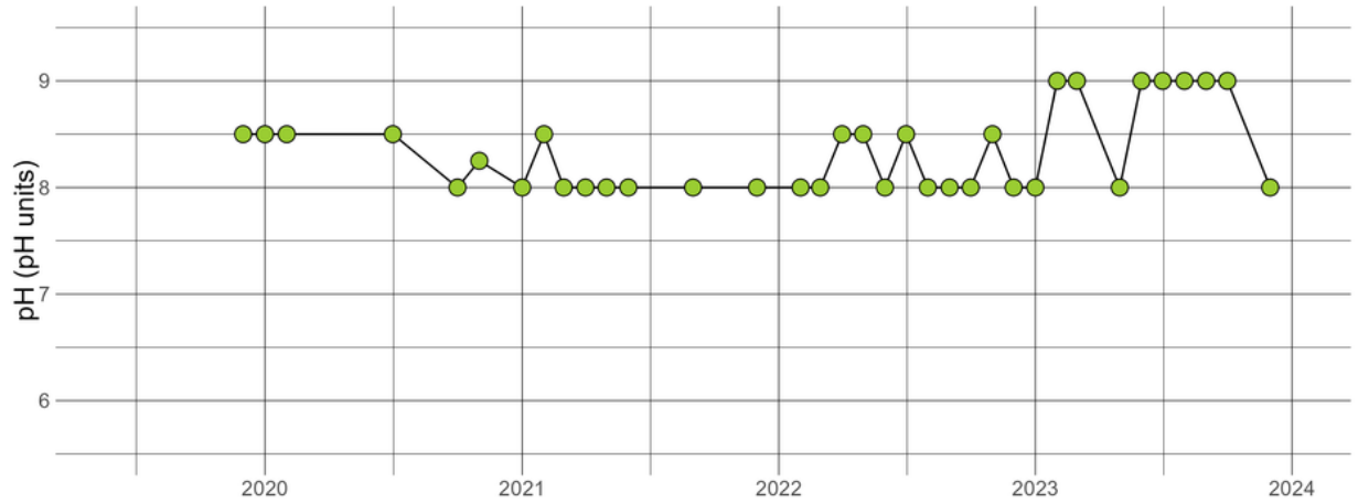
LITCONCRE12.56 - pH
