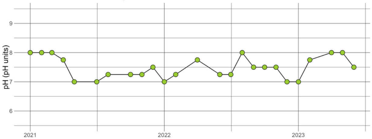
SOUBRACODCRE23.11 - pH
