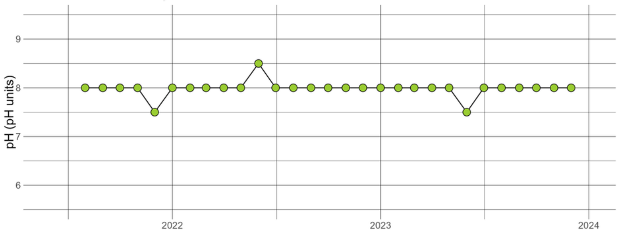
UNTCODCRE1.28 - pH
