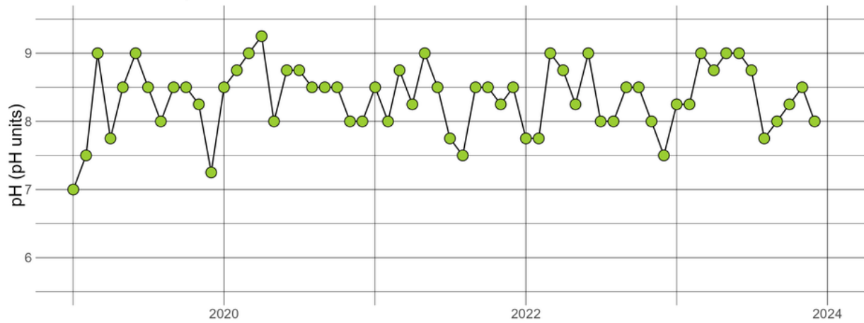
BERCRE1.22 - pH
