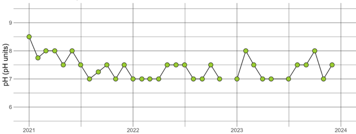
CODCRE5.77 - pH
